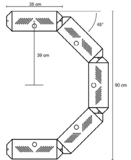
Minimaler Kurvenradius
